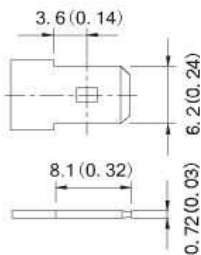
F2 Terminal
